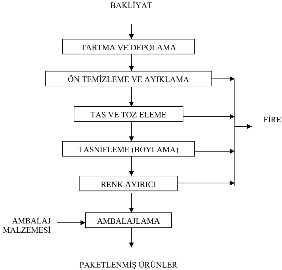
Şekil-1: Bakliyat İşleme Paketleme İş Akış Şeması
