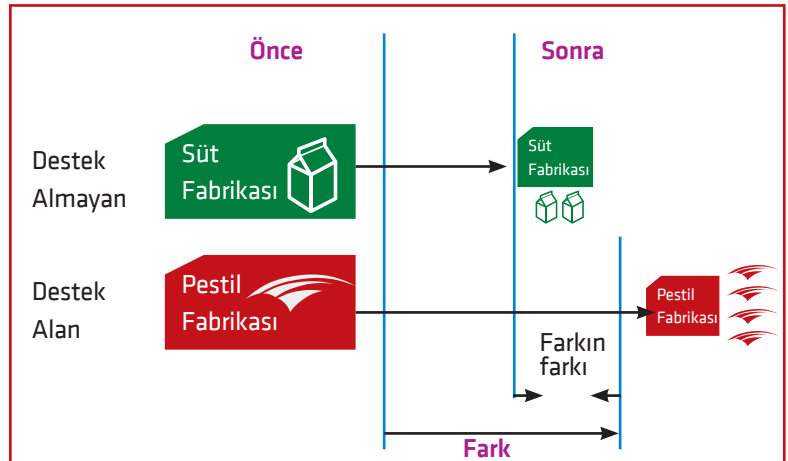
Şekil 1: Farkın Farkı Yöntemi
