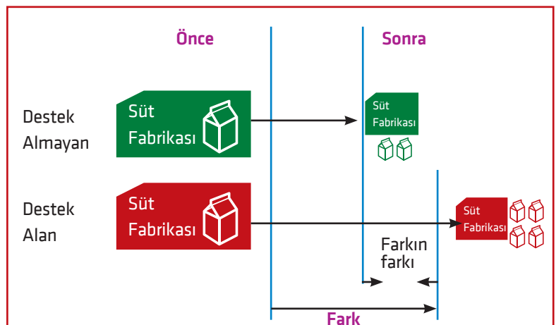
Şekil 2: Eğilim Skor Eşleşmesi Yöntemi
